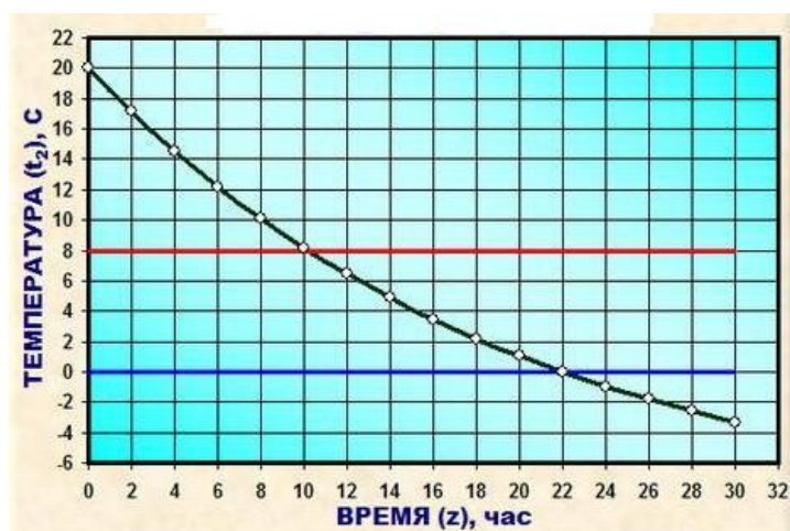
Рис. 1. Изменение температуры воздуха на объекте в зависимости от времени после отключения отопления при температуре наружного воздуха -10^{\circ}\text{C}
